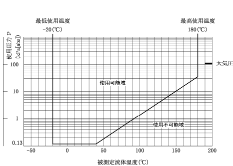
図2 使用圧力と接液温度
