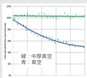
炭素の発光線(193nm)における、発光強度の経時的変化
