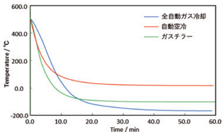
冷却ユニットの比較
