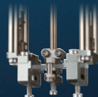
両持ち曲げ アタッチメント (兼片持ち曲げ)
