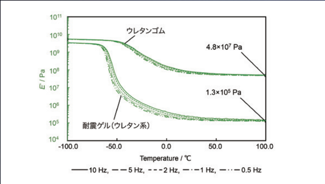
ウレタンゴムと耐震ゲル(ウレタン系)の比較
