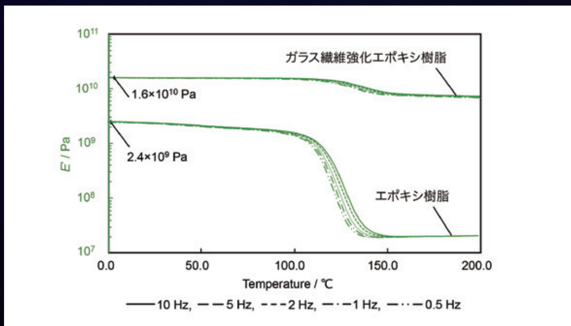
エポキシ樹脂とガラス繊維強化エポキシ樹脂の比較
