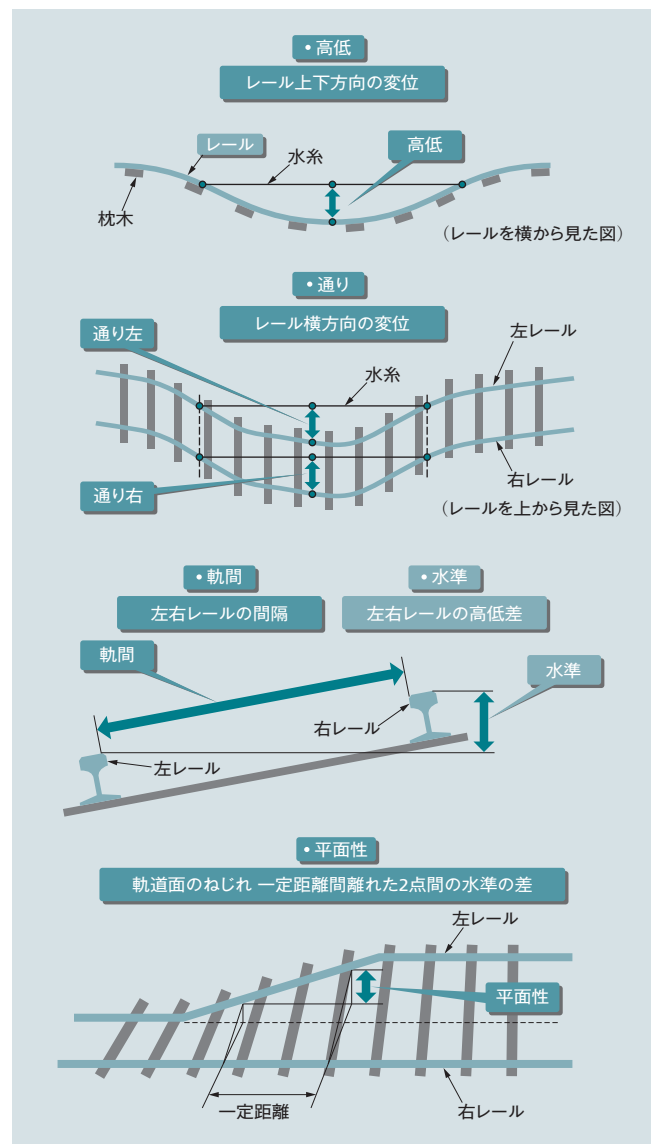
図1 | 軌道検測の測定内容 検測（検査測定）しなければならない軌道変位の概略を示す。
